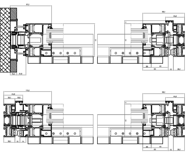
SECCIÓN B-B
