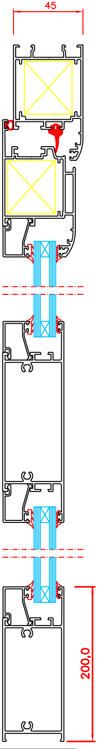
Sección Vertical B - B' Escala 1:1
